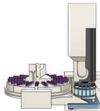
Agilent 7693 Autosampler
