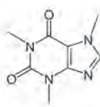
Caffeine
